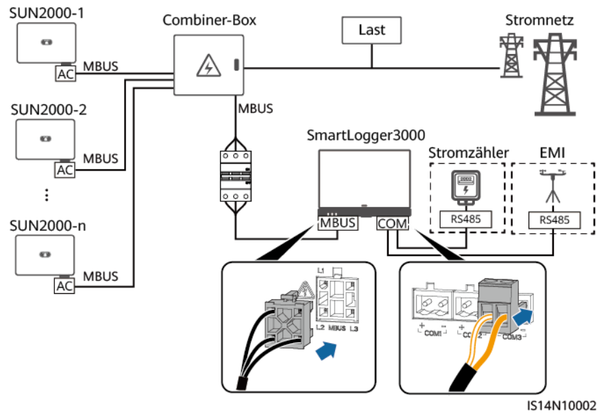
Abbildung 5-22 MBUS-Kommunikation (kommerzielle und industrielle Szenarien in China)
