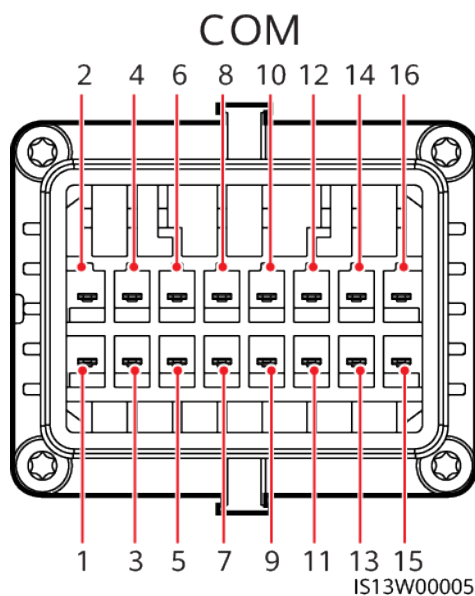
Abbildung 5-17 Pin-Definitionen
