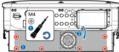
Abbildung 8-2 Schrauben von der Lüfterhalterung entfernen
