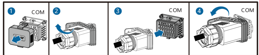
Abbildung 5-30 Sichern des Signalkabelanschlusses
