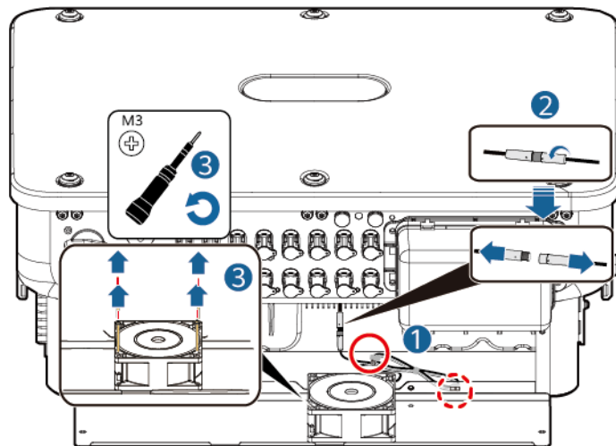
Abbildung 8-3 Entfernen eines defekten Lüfters
