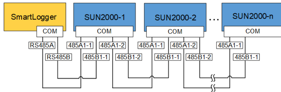
Abbildung 5-20 SmartLogger-Netzwerkaufbau
