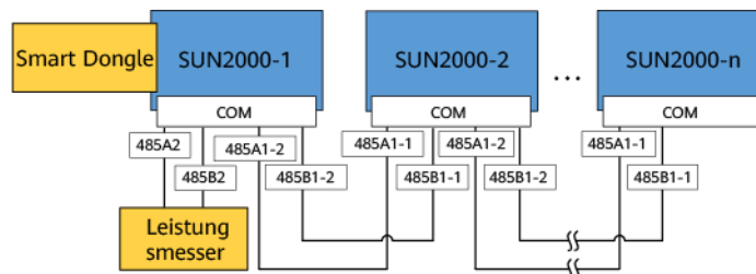
Abbildung 5-19 Smart Dongle-Netzwerkaufbau
