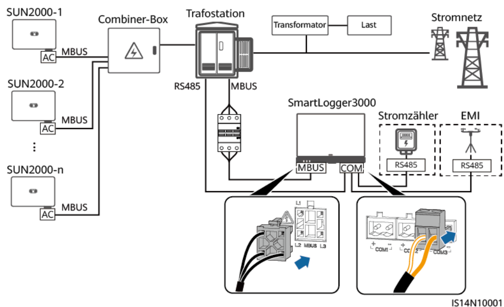
Abbildung 5-21 MBUS-Kommunikation (Großanlagen)
