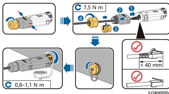
Abbildung 5-16 Anschließen eines WLAN-FE Smart Dongle (FE-Kommunikation)
