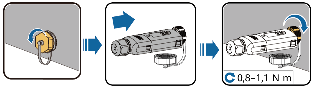
Abbildung 5-15 Anschließen eines WLAN-FE Smart Dongle (WLAN-Kommunikation)
