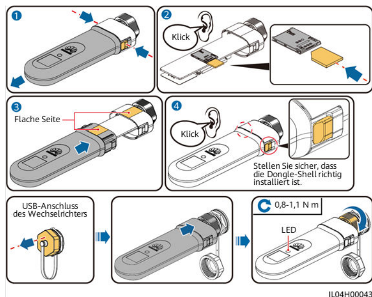
Abbildung 5-48 Anschließen eines 4G Smart Dongle (SDongleB-06)
